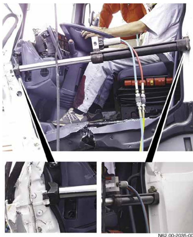
Entlastungsschnitte (Pfeile)
