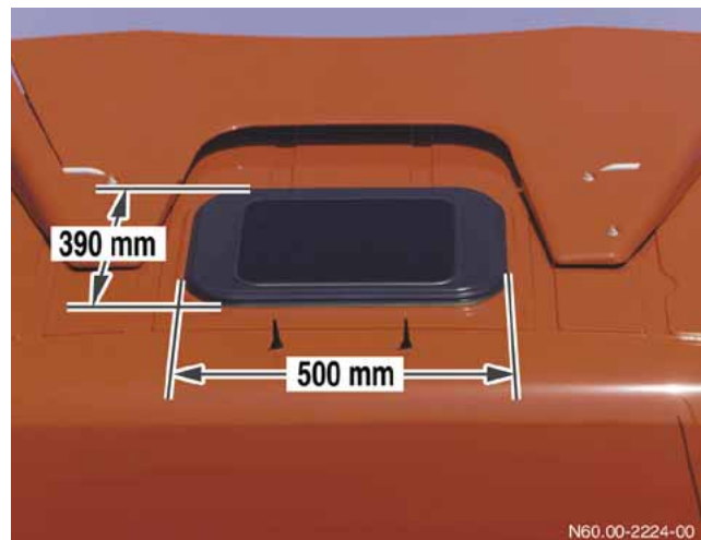
Zugangsmöglichkeit Dachluke
